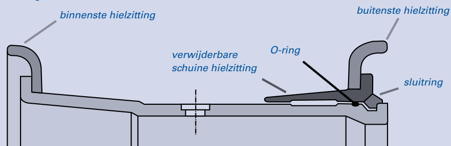
Afb. 11: meerdelig wiel in onderdelen
