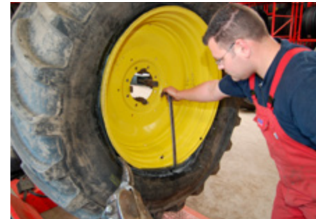
Afb. 8: eerste hiel verwijderen
