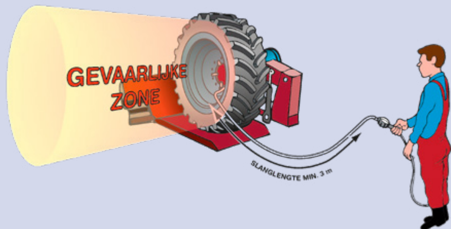
Afb. 46: oppompen buiten bandenkooi op een montageapparaat
