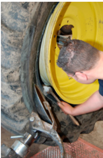
Afb. 7: insmeren met montagepasta
