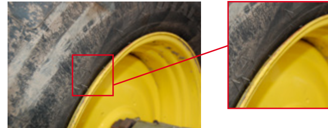
Afb. 37: hiel nog niet volledig gezet bij 1 bar voorspanning
