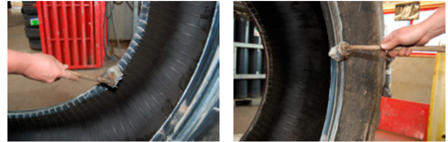
Afb. 15 + 16: hiel binnen en buiten insmeren
